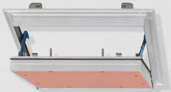
TRAPPE COUPE FEU PLAFOND 90 MN - 40 MM 2 PLAQUES DE 20 MM • CERTIFICAT EI 90
