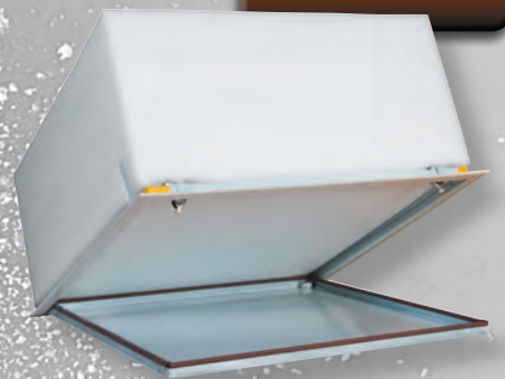
KIT TRAPPE ISOLANTE ET ETANCHE R8 (R=8.13)
